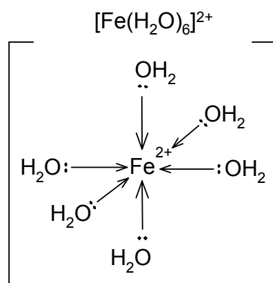
Hexaaquairon(II) ion
