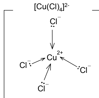
Tetrachlorocuprate(II) ion
